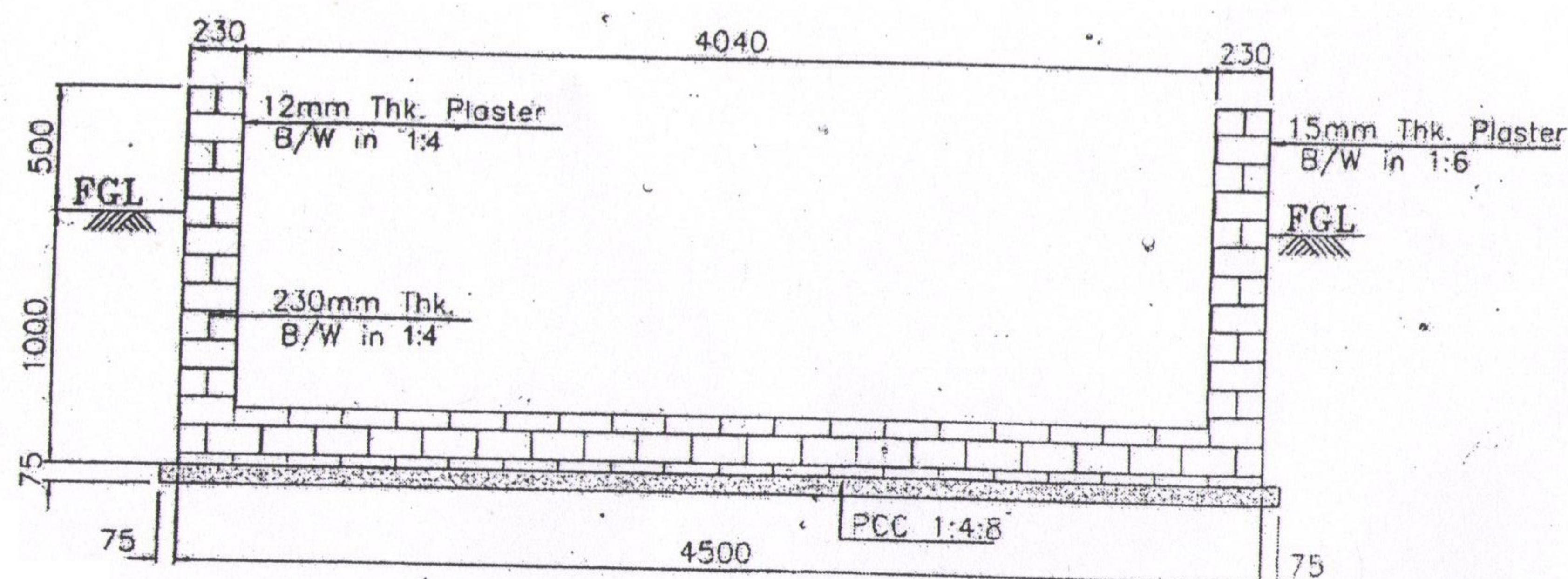
SECTION A-A
